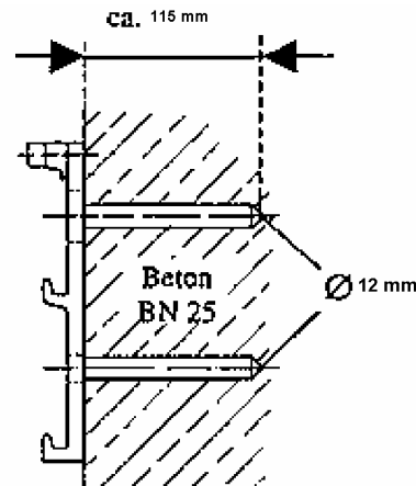
Bild 1b Wandmontage
